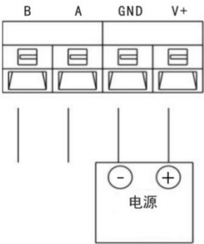
RS485输出
