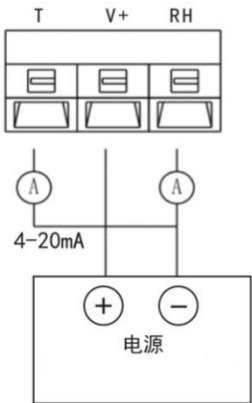
电流输出
