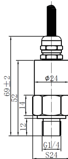
带标准电缆直出线
