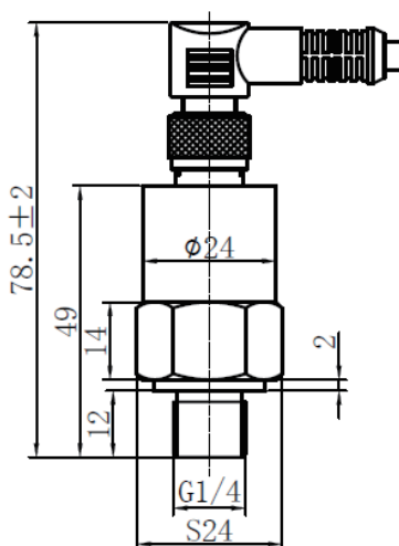
带 M12*1 圆形航空插头
