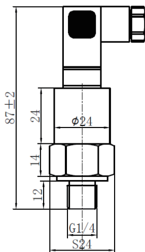
带小赫斯曼接头
